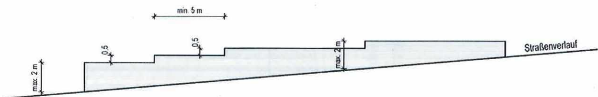
Schemaschnitt Mauerkrone
