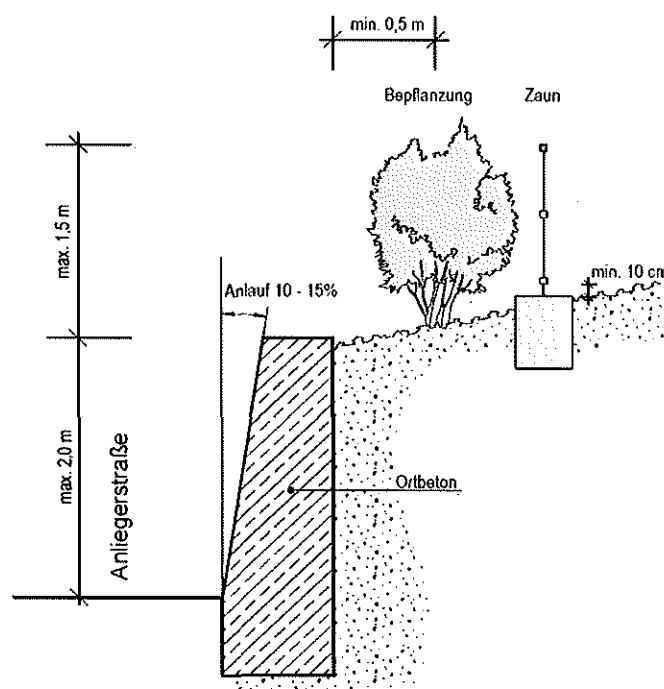
Schemaschnitt Stützmauern
