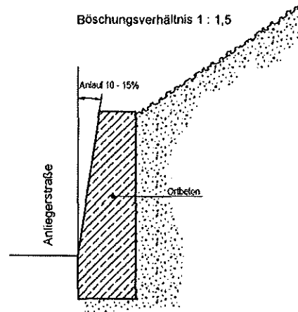
Schemaschnitt Böschungsverhältnis
